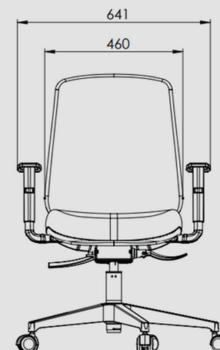
Mecanismo Back System 10.2 permite a regulação de altura através de alavanca (direita) e regulação de inclinação do encosto com travamento na posição desejada através de alavanca (esquerda).
